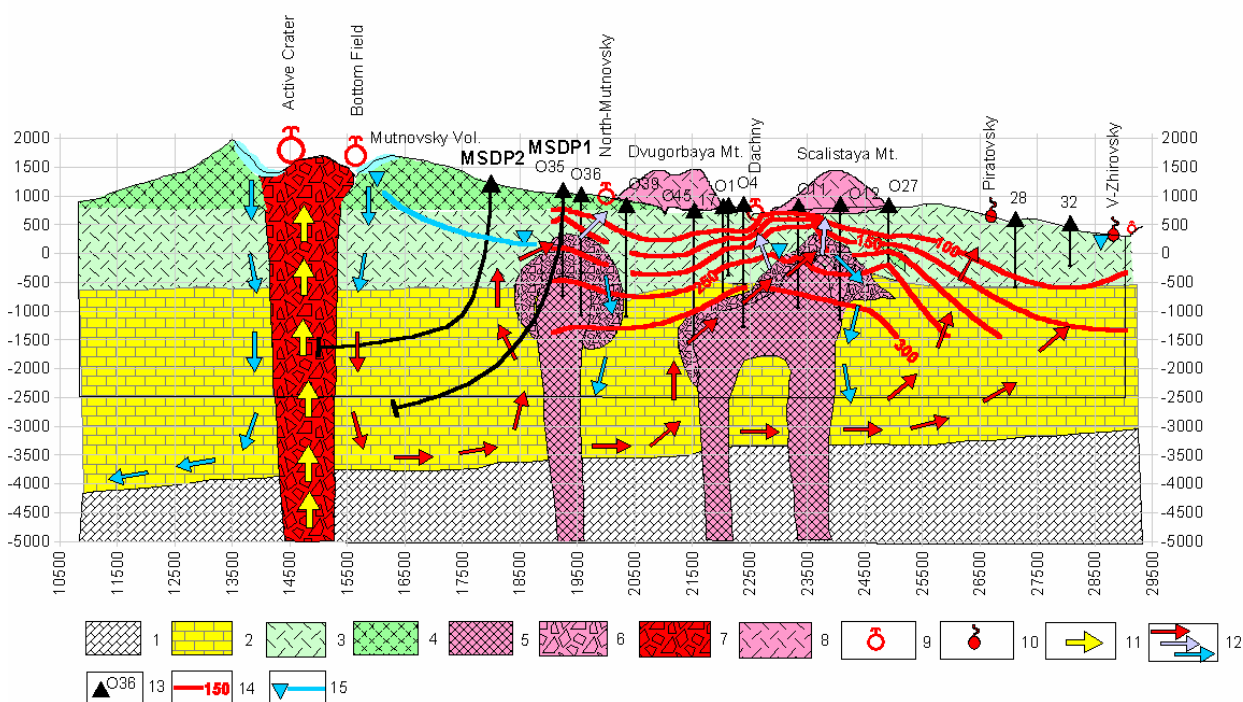
Рис.1. Гидрогеологический разрез и концептуальная модель Мутновского вулкана и Мутновского геотермального месторождения: 1 – Кристаллический фундамент, 2 – Меловой фундамент и миоценовые песчаники, 3- Неогеновые вулканогенно-осадочные породы, 4 – Мутновский стратовулкан (Q 3 -Q 4 ), 5 – Диоритовые интрузии, 6 – Диоритовая контактовая зона, 7 – Магматическая система Мутновского вулкана, 8- Кислые экструзии (Q 3 -Q 4 ), 9- Фумарольные поля, 10 – Горячие источники, 11- Магма и магматические флюиды, 12 – Гидротермальные флюиды, 13 – Геотермальные скважины, 14 – Распределение температуры (Мутновское геотермальное месторождение), 15 – Уровень подземных вод в Мутновской гидротермальной системе, м. абс.
