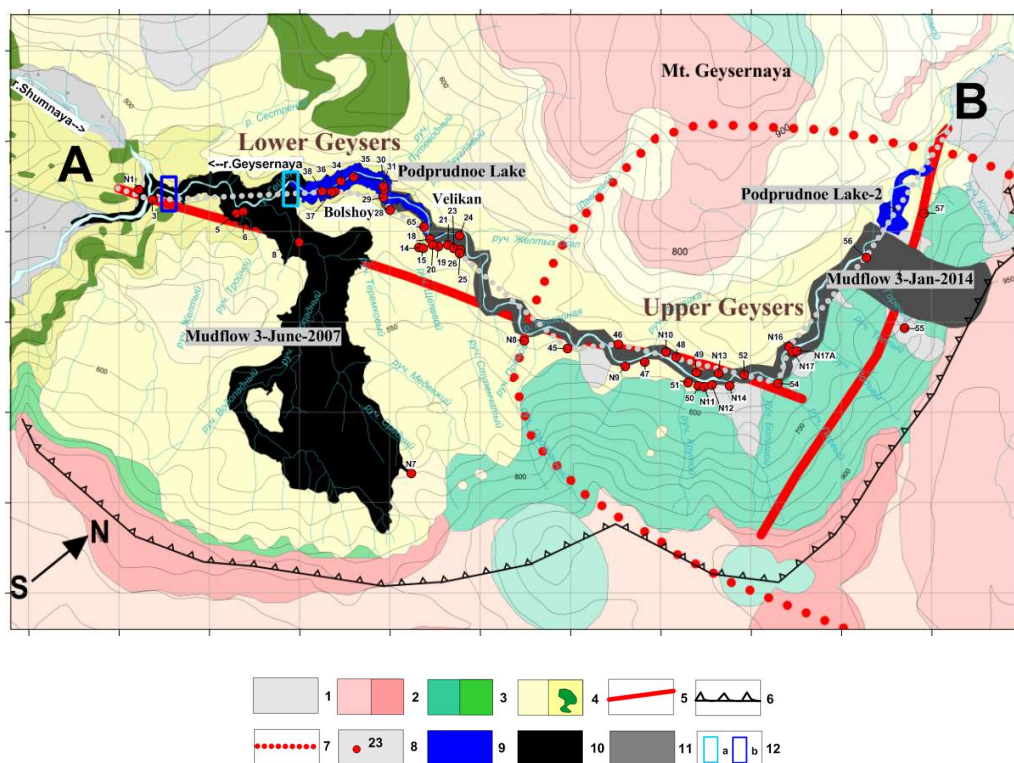
Рис. 4. Схематическая карта Долины Гейзеров. Легенда: 1 – аллювиальные и ледниковые отложения Q 3-4 ; 2 – проницаемые блоки риолитовых, дацитовых и андезитовых экструзий ( \alpha\xi Q_3^4 ); 3 – базальтовые, андезитовые, и дацитовые лавы и пирокластика ( \alpha Q_3^{1-2} ); 4 – блоки низко проницаемых кальдерно-озерных отложений (Q 3 4 ), осложненные комплексом даек (Q 3 3ust ); 5 – предполагаемые термовыводящие разломы; 6 – граница Узон-Гейзерной депрессии; 7 – возвышенная область, связанная с предполагаемым контуром активного магматического резервуара (Lundgren et al., 2006); 8 – гейзеры и горячие источники (нумерацию см. в таблице 6 в работе Kiryukhin, 2016); 9 – Подпрудное озеро и Подпрудное озеро-2, сформированные оползнем и селем; 10 – катастрофический оползень-сель 3.06.2007; 11 – оползень-селевой поток 3.01.2014; 12 – точки измерения расхода реки Гейзерной: а – выход из Подпрудного озера, б – в устье р. Гейзерной. Размерная сетка – 500 м.
