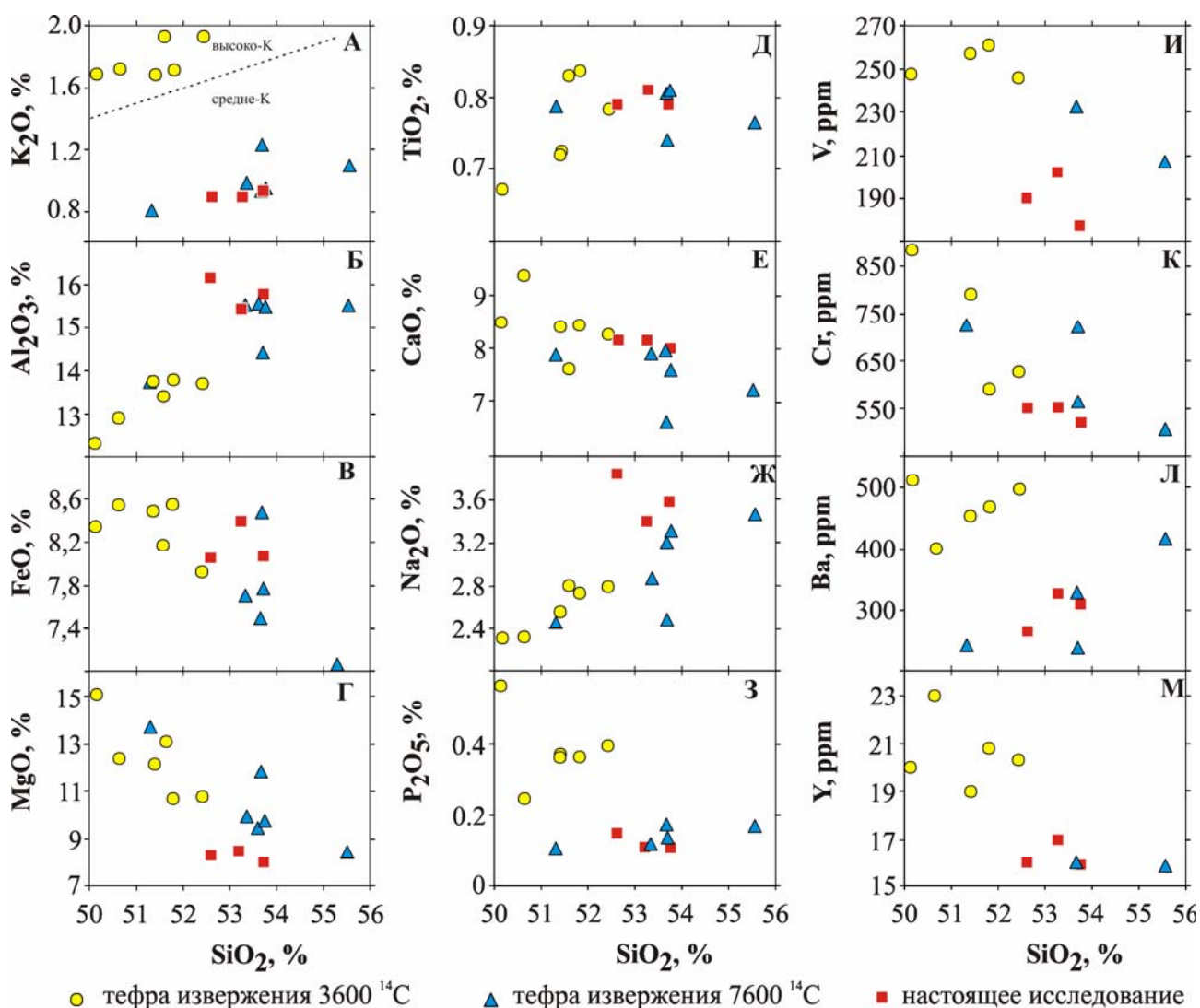
Рис. 3. Зависимость содержания макро- и микроэлементов от кремнезема в тефре извержений 3600 и 7600 14 С л.н. [Ронотарева et al., 2007], а также в найденных коренных базальтах.
