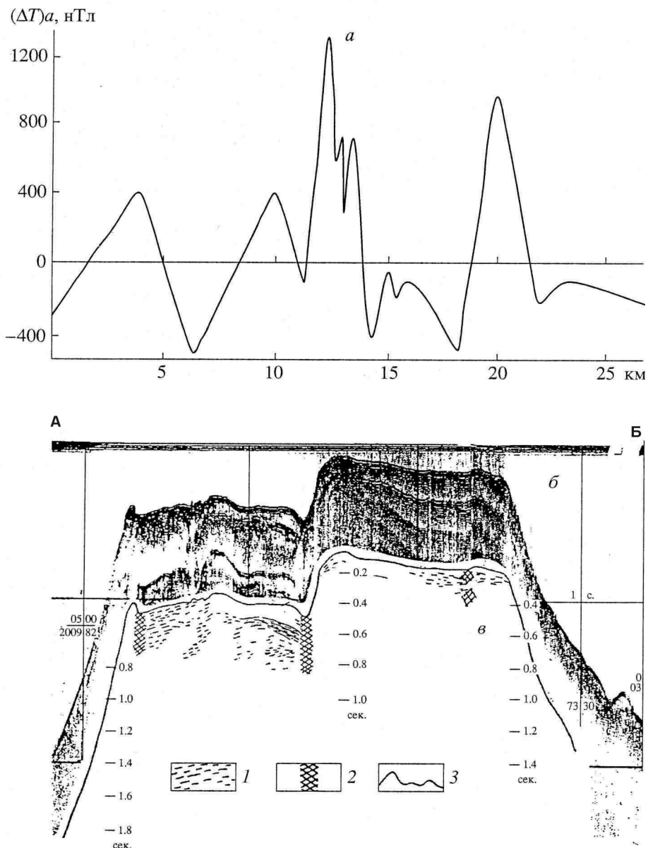
Рис. 3. Изменение аномального магнитного поля (а), фрагмент сейсмограммы НСП (б) и временной разрез (в) по профилю А-Б. 1 – отражающие границы; 2 – кальдерообразующие разломы; 3 – выходы «акустического фундамента». Положение профиля см. на рис. 2.
