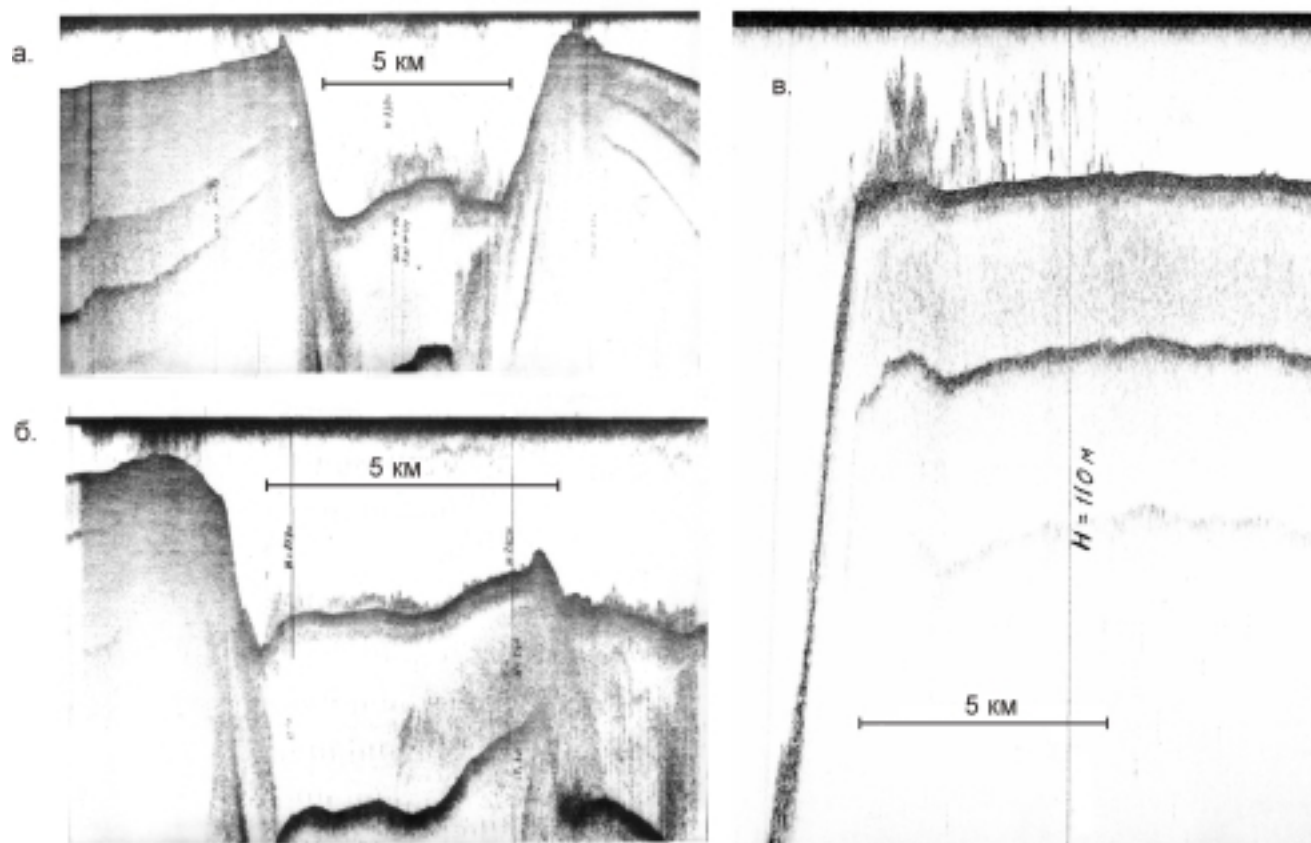
Рис. 5. Акустические помехи в водной толще вулканического массива Черных Братьев, зафиксированные на самописце эхолота WD-110М, центральная частота 12.5 кГц.
