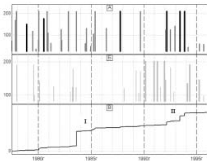
Рис. 3. Распределение во времени землетрясений 1977 – 1995 гг., вызвавших различный тип отклика в изменении дебита источника: а – землетрясения, вызвавшие повышенный (черные вертикальные линии) и нормальный (темно-серые вертикальные линии) отклик дебита источника; б – землетрясения, вызвавшие пониженный отклик источника (толстые серые вертикальные линии) и землетрясения, не вызвавшие изменения дебита (тонкие серые линии); в – кумулятивный график выделения сейсмической энергии радиусе до 450 км от п. Пиначево. I – сейсмическая активизация 1983-1984 гг., II – сейсмическая активизация 1992 -1993 гг.
