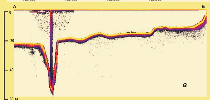
Рис. 6. Результаты батиметрической съемки озера Горячее: а - гипсометрическая модель; б - батиметрическая схема, изобаты проведены через 5 м.; в - эхолотный профиль по линии АБ.
