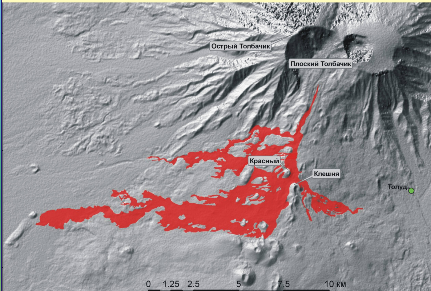
Рис. 1. Схема распространения лавовых потоков по состоянию на конец марта 2013 г. Схема построена на основе дешифрирования спутниковых снимков TERRA ASTER (NASA, JPL) в EO-1 ALI (NASA). Топографическая основа SRTM X-band. Составил Д.В.Мельников.
